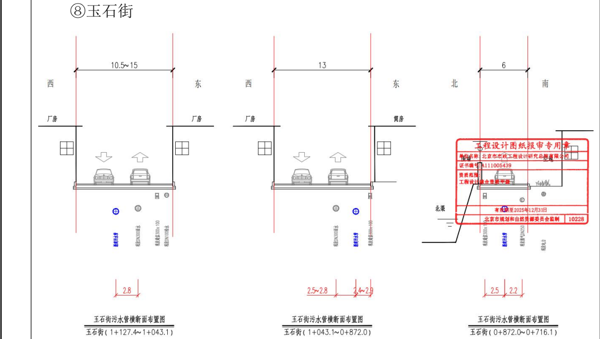
图 2.4-12 玉石街横断面图设计图
