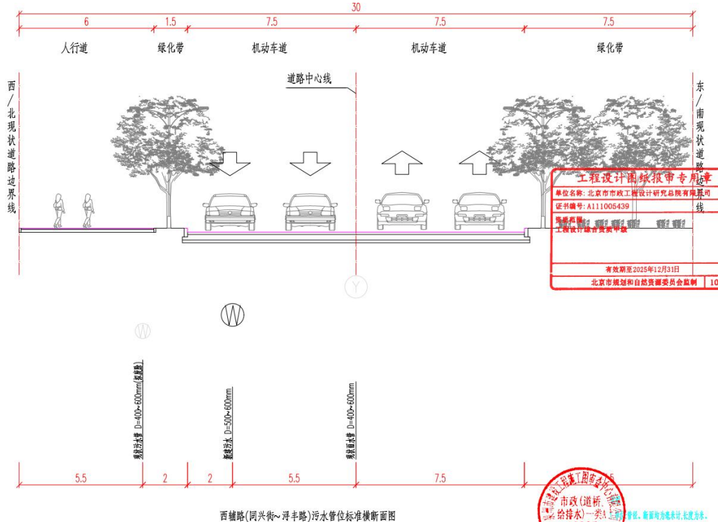
图 2.4-8 西辅路（同兴街～浔丰路）横断面图设计图
